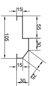
DOORSILL INOX
