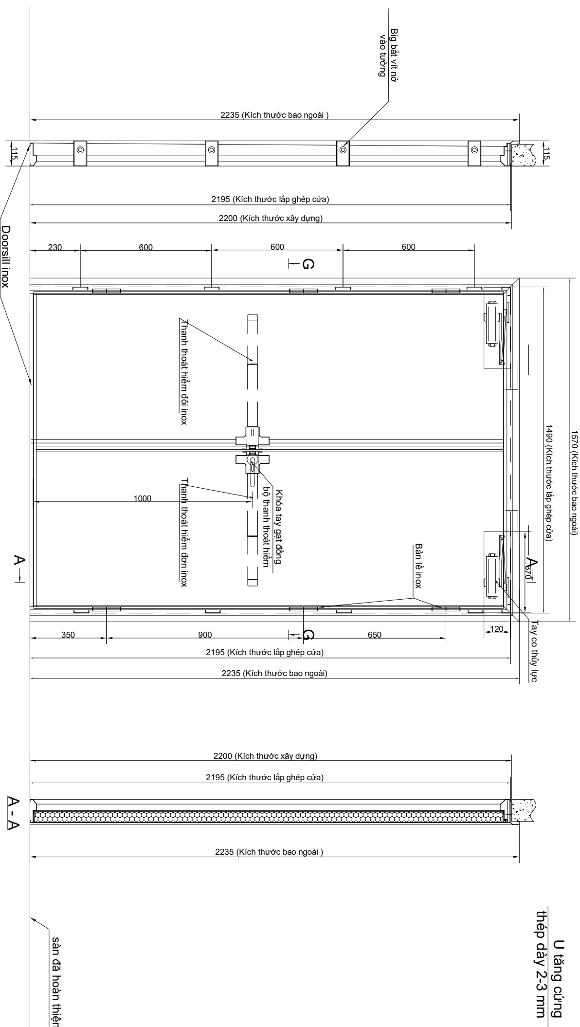
MẶT CẮT KHUNG CỬA
