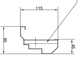
MẶT CẮT KHUNG CỬA
