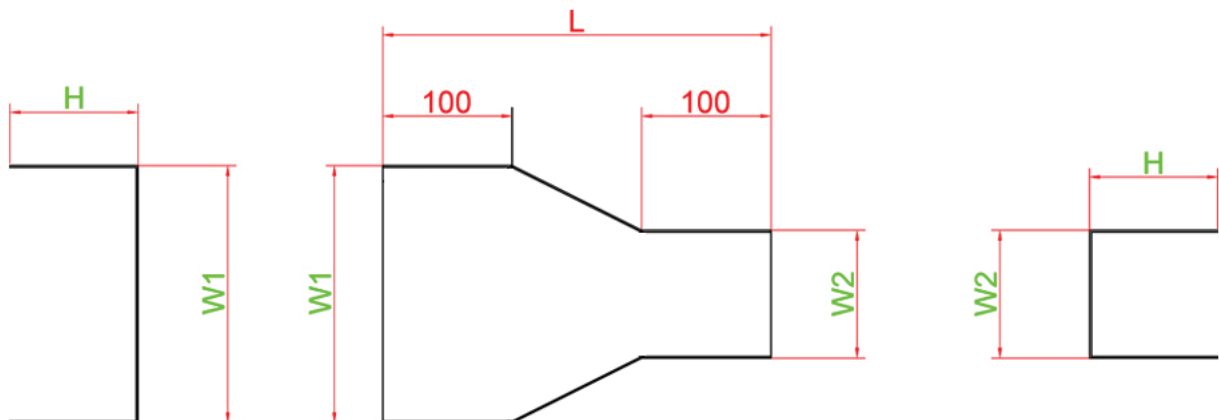
BẢN VẼ TĂNG/ GIẢM MÁNG CÁP
